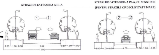
PROFILURI TRANSVERSALE CARACTERISTICE PENTRU DRUMURILE PROPUSE PE TRASEE NOI SI PENTRU REABILITARE cote minime
